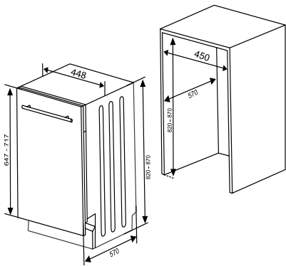
BSV45-8.1, BSV45-9BS.1
