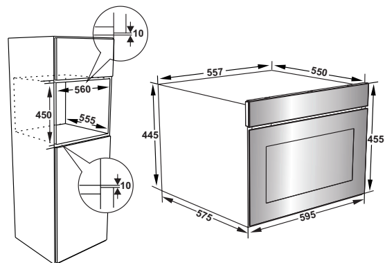
BCB45-10BL, BCB45-161BL
