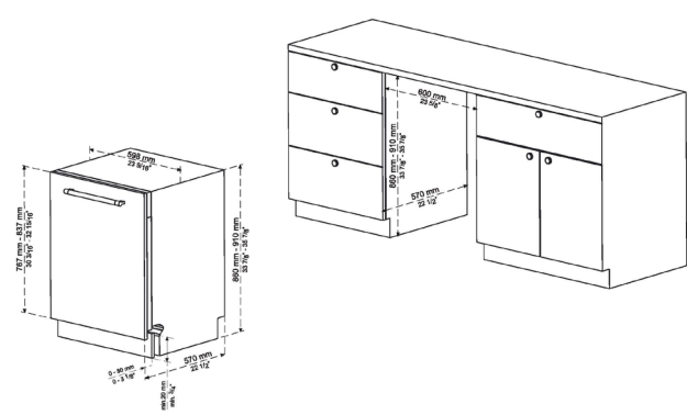
BSV60-9.2-TT-SD
