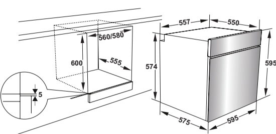
BSV60-9.2-TT-SD
