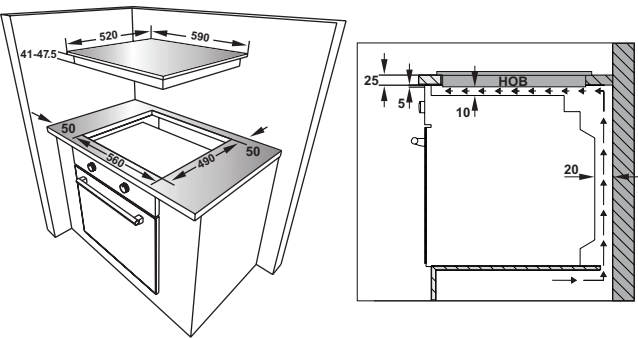
BSV45-8.1, BSV45-9BS.1
